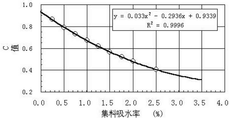
图 B.5.3 计算集料有效相对密度的权重系数 C 值
