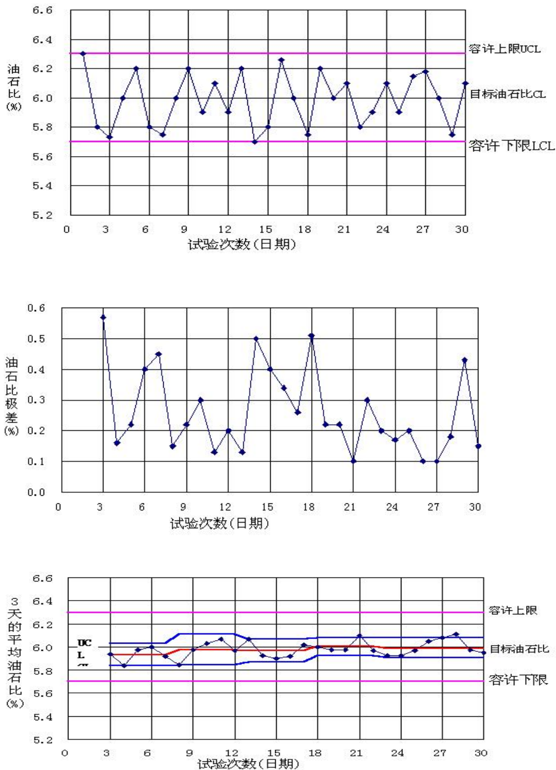
图 F.0.3 动态质量管理图 ( \bar{X}-R 管理图) 示例 (油石比, %)
