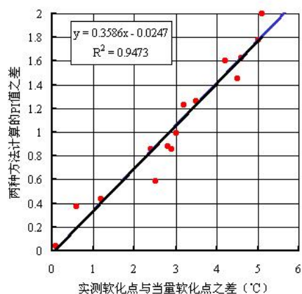
不同软化点测定方法与PI值计算结果的关系
