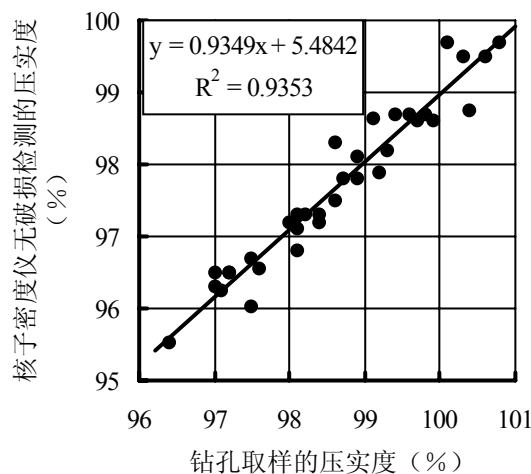
图 11.4.8-1 核子仪与钻孔试件结果的标定关系
