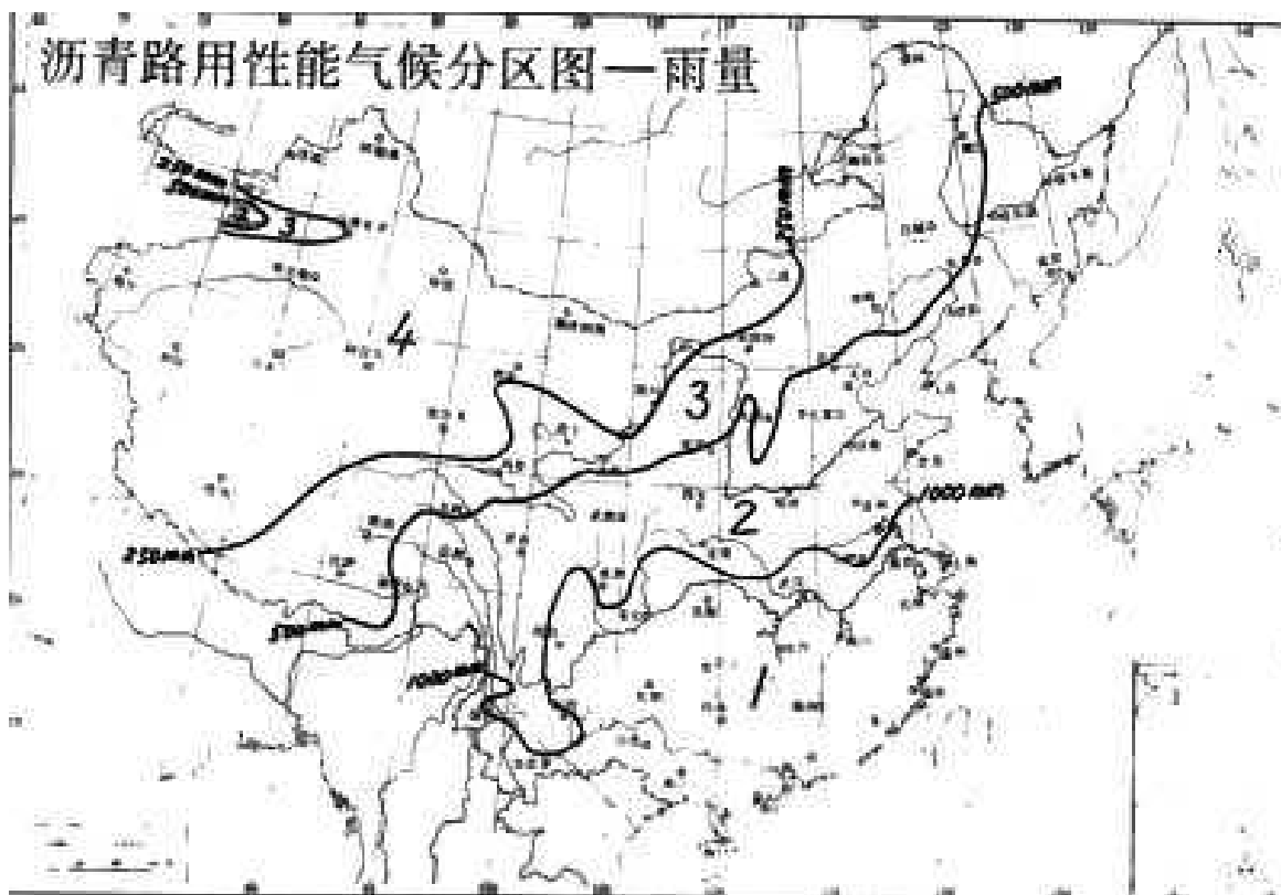
图 A. 4. 6-2 中国沥青路面气候分区图(雨量)
