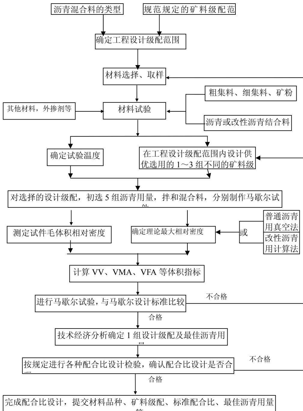
图 B. 1. 3 密级配沥青混合料目标配合比设计流程图
