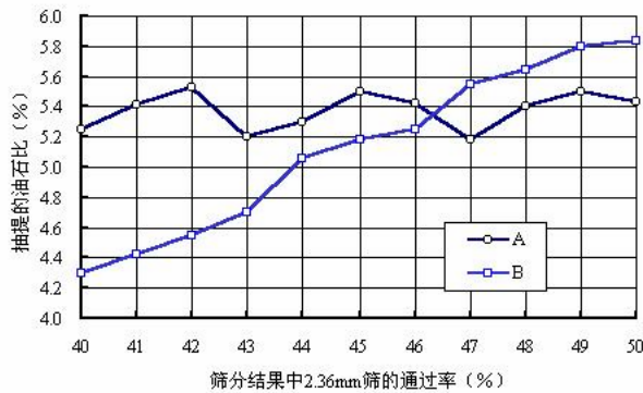
图 F.0.1 关键性筛孔 2.36mm 通过率与油石比变化的关系
