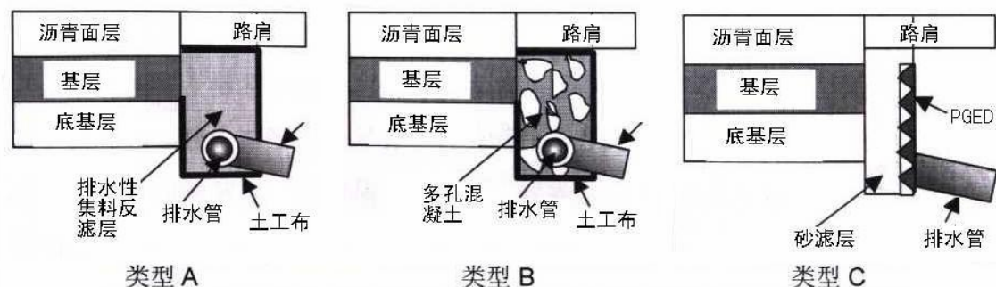
图 10.7.1 AASHTO 沥青路面结构层边缘排水方案
