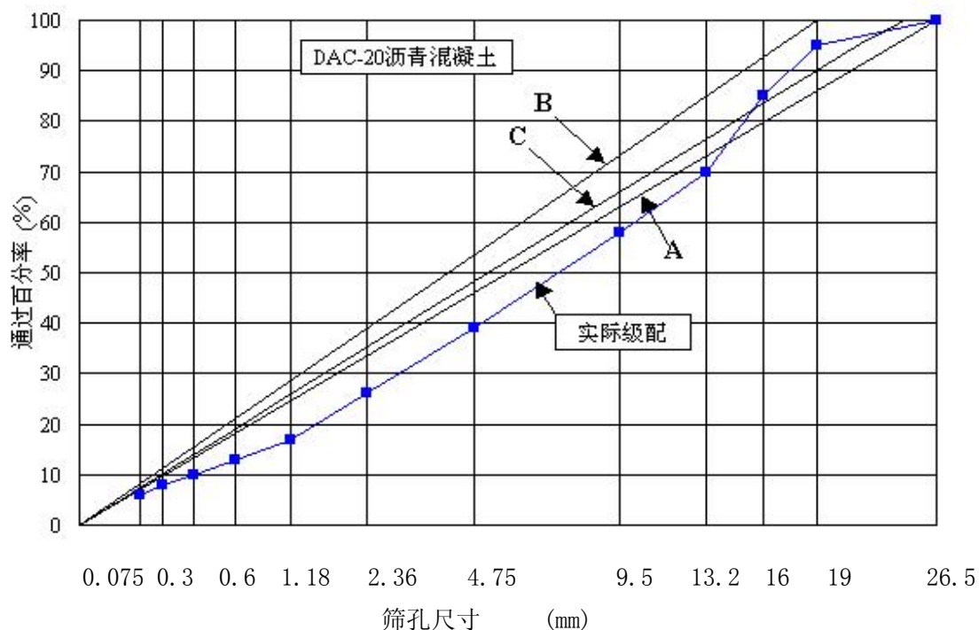
图 B.4.2 AC-20 沥青混合料矿料级配最大密度线的 3 种不同画法
