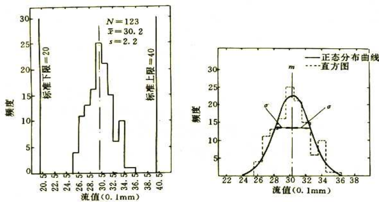
图 F.0.3-2 工程质量指标检测结果的直方图及正态分布曲线示例
