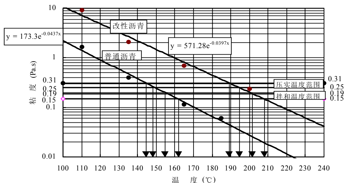
图 5.2.4 普通沥青及改性沥青的粘温曲线
