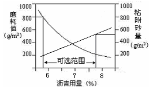
图 6.5.7.4 确定稀浆封层和微表处最佳沥青用量的曲线
