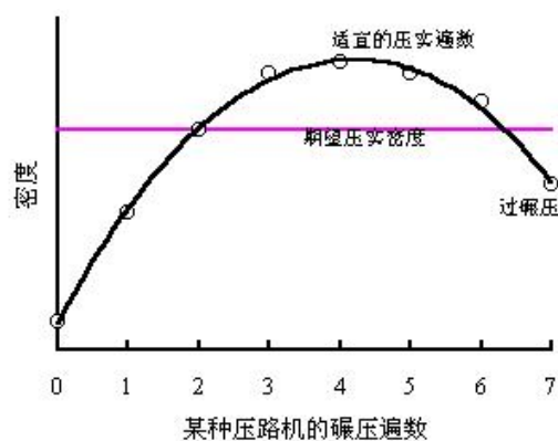
图 11.4.8-2 沥青路面的过碾压
