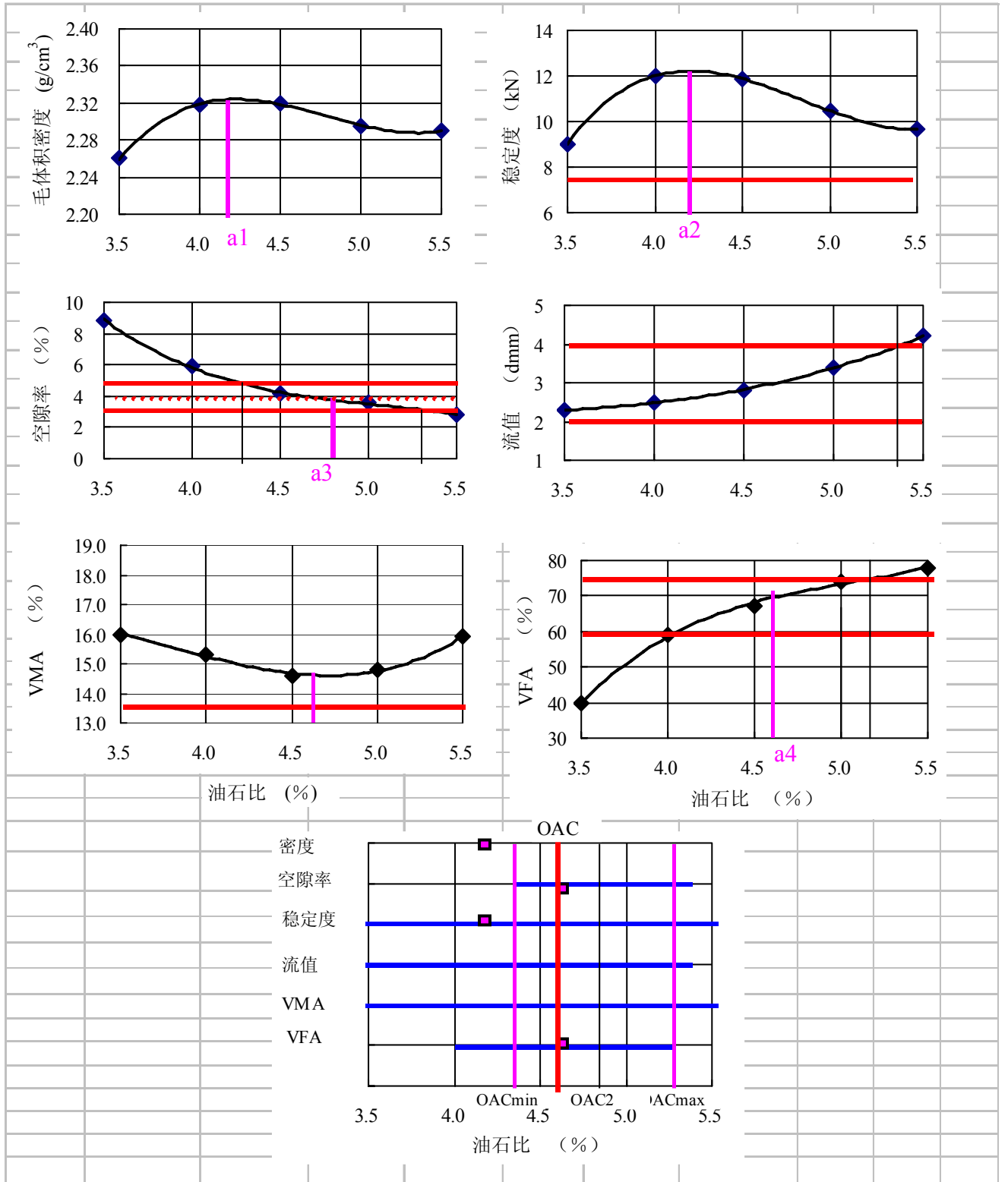
图 B. 6. 1 马歇尔试验结果示例
